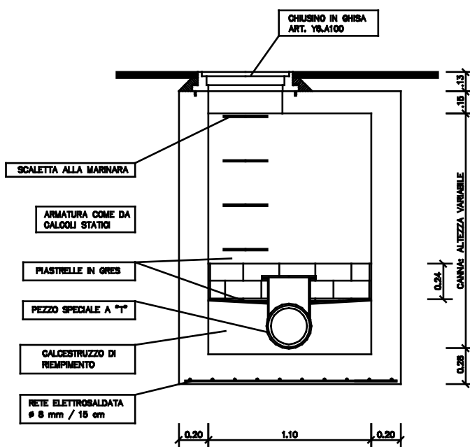
E.1.10.91 POZZETTI DIM 1.10 x 1.10 PER CONDOTTE IN PRESSIONE SEZ. A-A SEZIONE A-A
